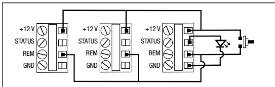
Abb. CDrei für Kurzschaltung konfigurierte PS-8RE III-Einheiten mit LED-Anzeige.
