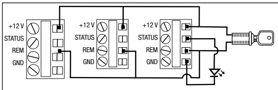
Abb. BDrei für Paralleldauerschaltung konfigurierte PS-8RE III-Einheiten mit LED-Anzeige.
