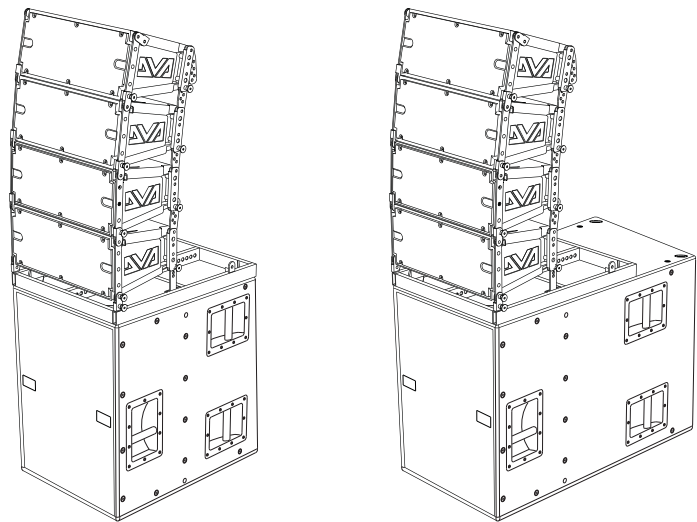
In appoggio con flybar (opzione DRK 10 oppure DRK 20) Groundstack with flybar (DRK 10 or DRK 20 option)
